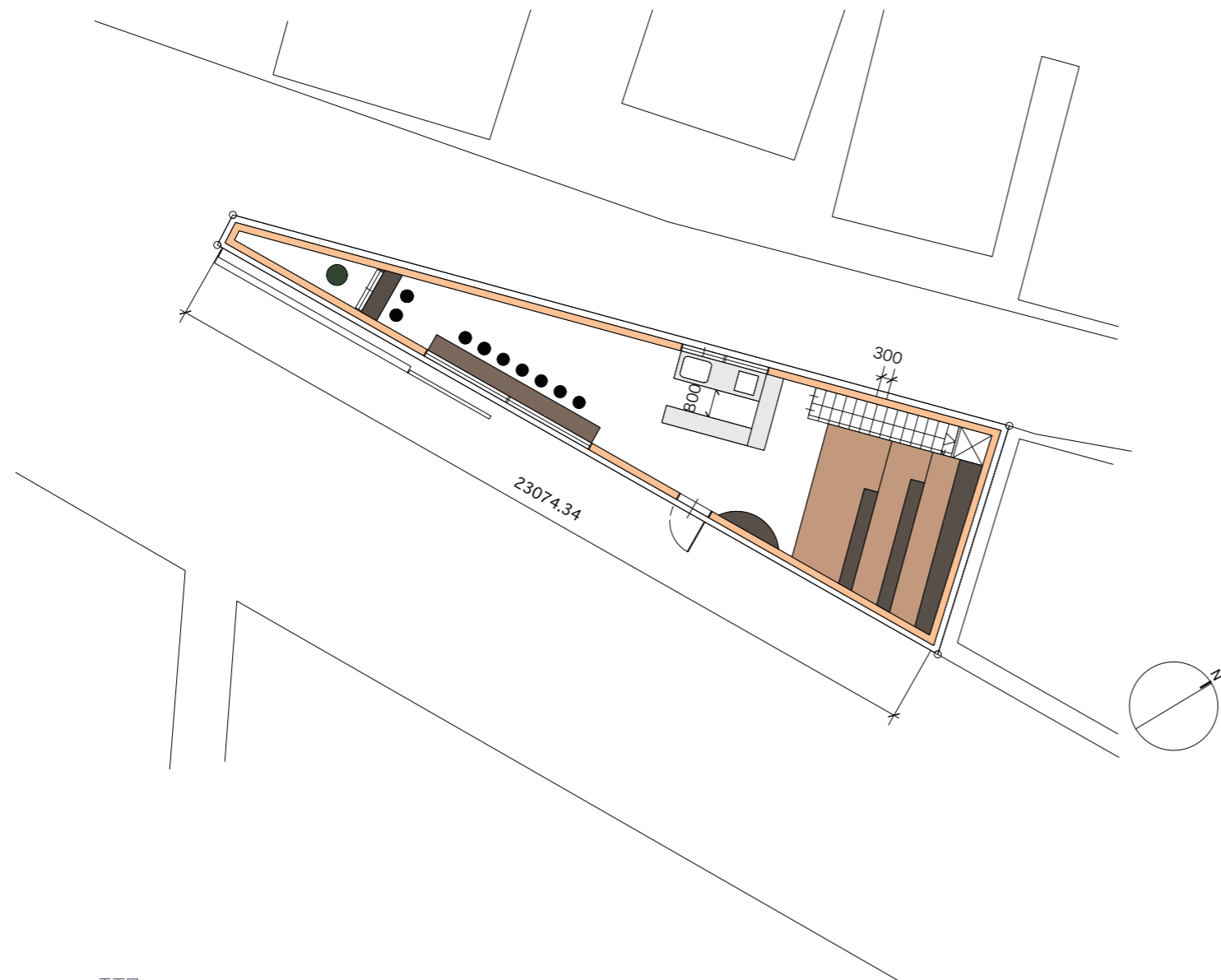
平面図
