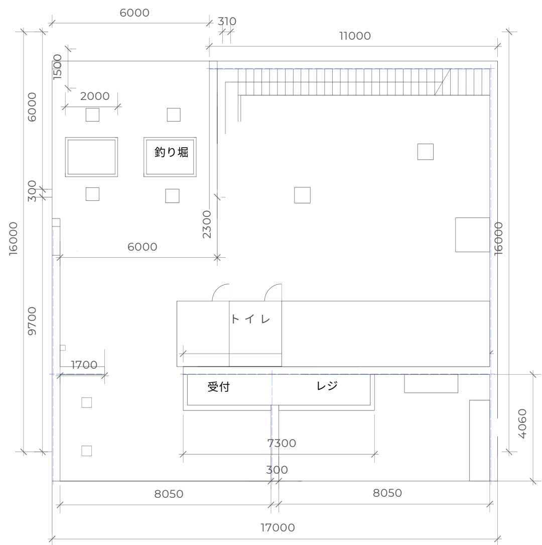
1階平面図 1/100
